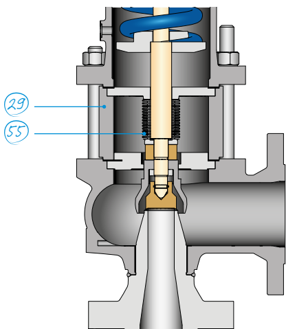
Bellows design Si 6405
