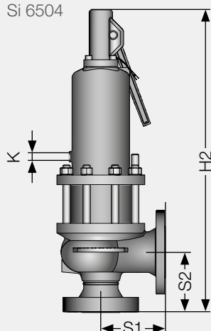
Si 6404 Si 6504
