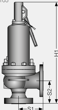
Si 6305 Si 6105
