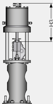
Actuator AK
