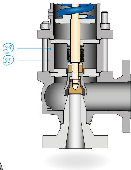
Bellows design Si 6403
