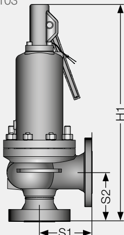
Si 6303 Si 6103
